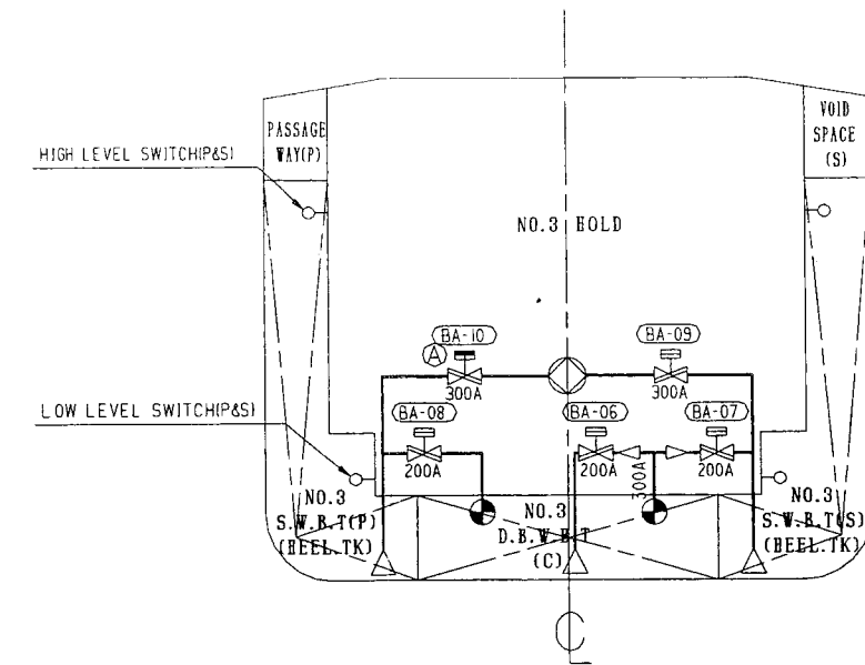
A-A SECTION
